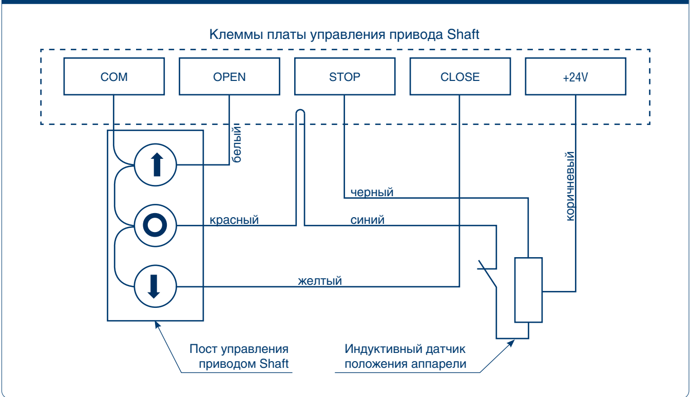
Рис. 5.5. Схема подключения индуктивного датчика положения аппарели для блока DCUT-2*
