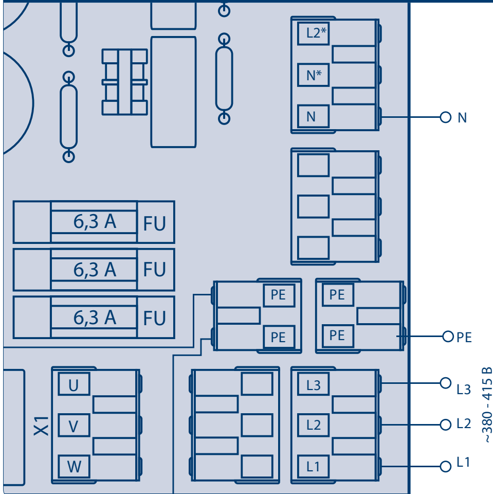
Рис. 5.2.1. Вид А. Подключение источника питания
